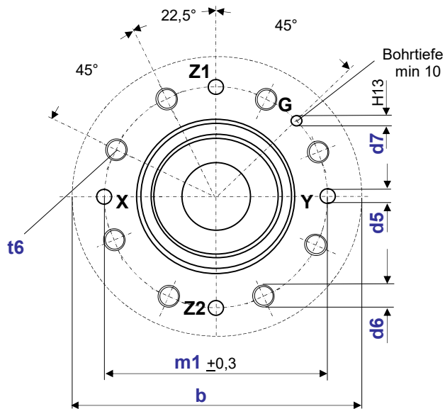
Abmessungen DIN 24342, DN80-100
