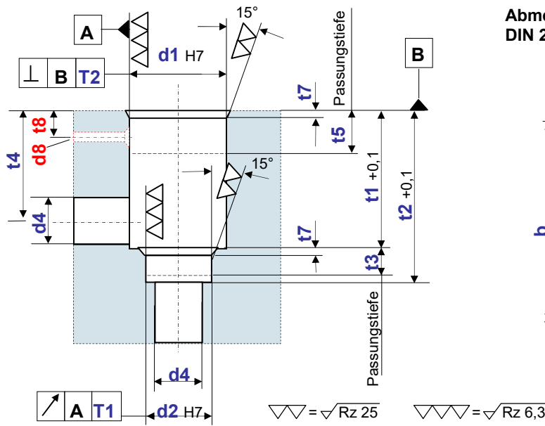
Abmessungen DIN 24342, DN80-100
